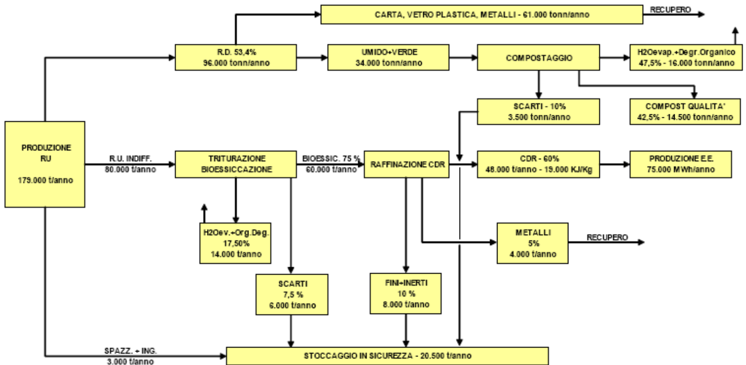
Fig. 20 - Soluzione B: schema di trattamento con bioessiccazione e produzione CDR (scenario anno 2014)
