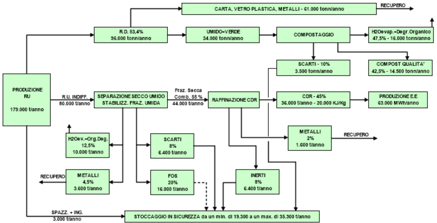
Fig. 19 - Soluzione A: schema di trattamento con separazione secco/umido e produzione CDR (scenario anno 2014)
